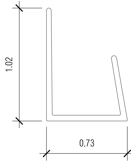
1 SIDE VIEW scale: 2:1
