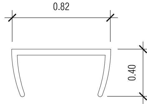
1 SIDE VIEW scale: 2:1
